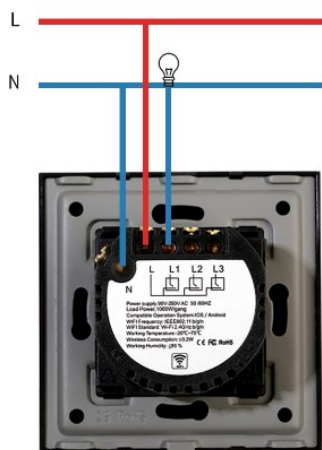
1 pav. Pagrindinio jungiklio prijungimo schema
