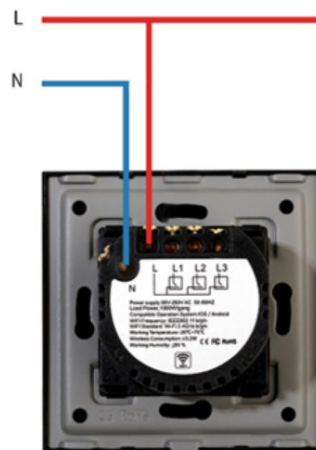
2 pav. Kito (nepagrindinio) jungiklio prijungimo schema
