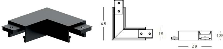
CORNER 90° HORIZONTAL (23131)
