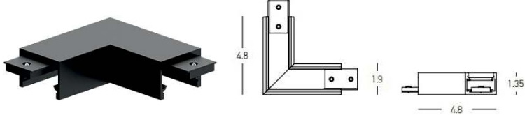
CORNER 90° HORIZONTAL (23131)
