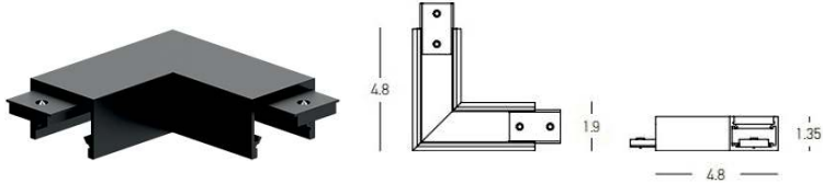
CORNER 90° HORIZONTAL (23131)
