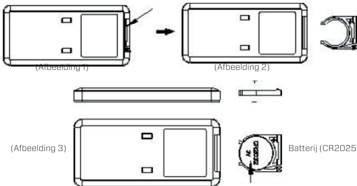
Afstandsbediening
